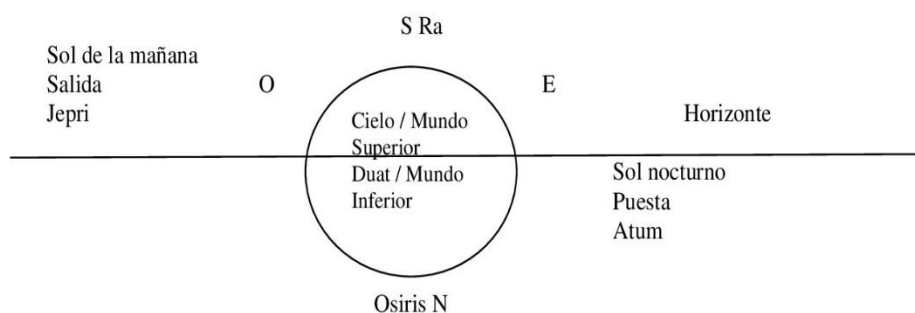
Esquema N°1: Modelo-base de la ciclicidad solar y su recorrido Wiebach-Koepke (1997,337)
